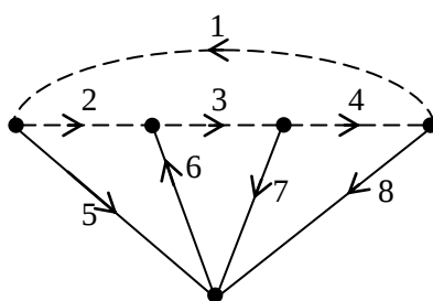
4.4-сурет. Электр тізбегінің граф бөлігі (подграф): тал (сызықтар) және байланыс тармақтары (үзік-үзік сызықтар)
