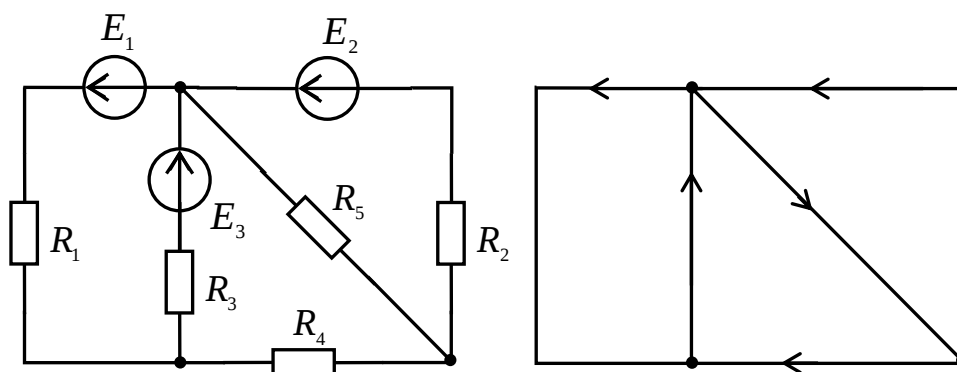
4.1-сурет. Электр тізбегі және оған сәйкес граф
